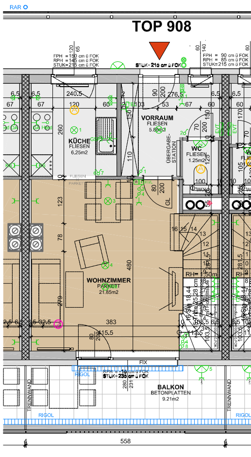
2. Obergeschoss
