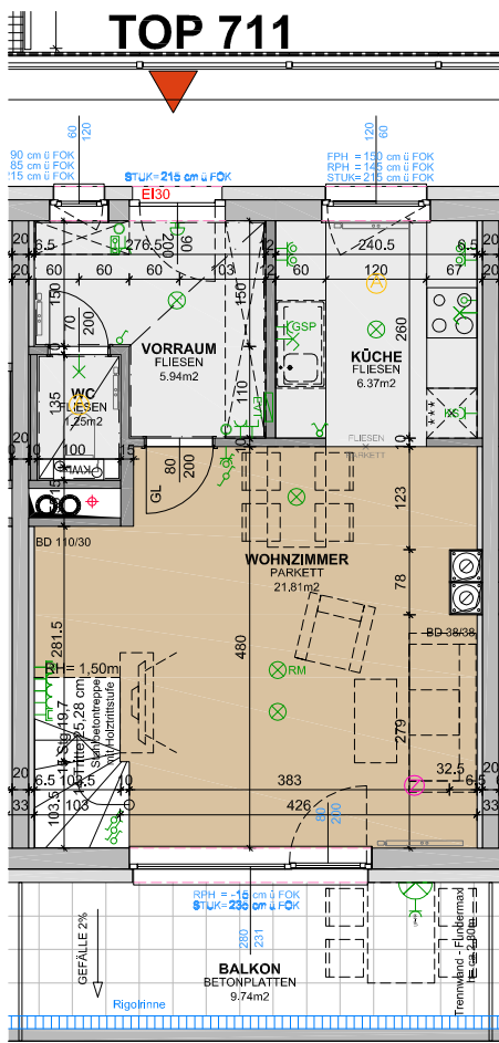
2. Obergeschoss
