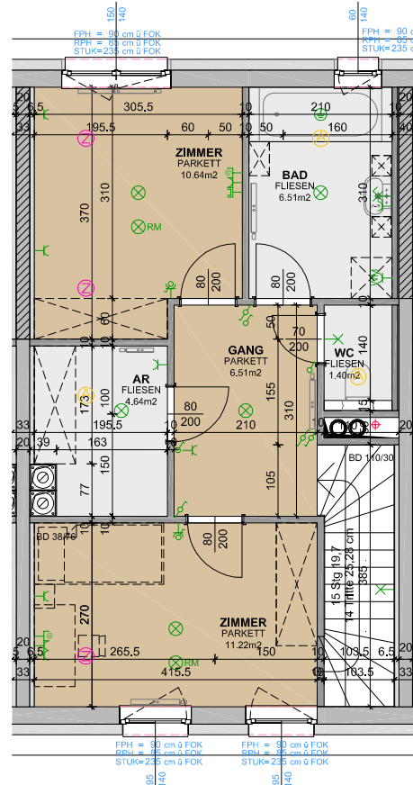
3. Obergeschoss
