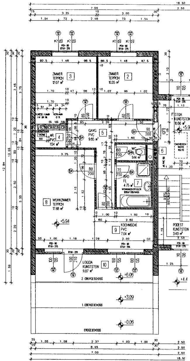
GRUNDRISS 2.OBERGESCHOSS
